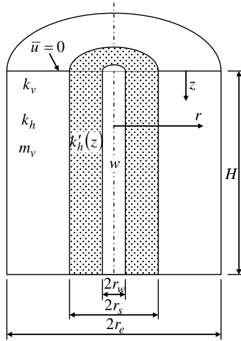
Fig. 1. Unit cell
