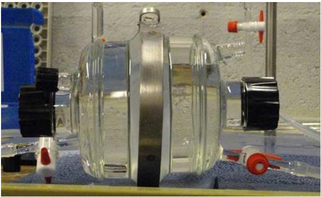
Diffusion cell (After Touze-Foltzet al,2012)
